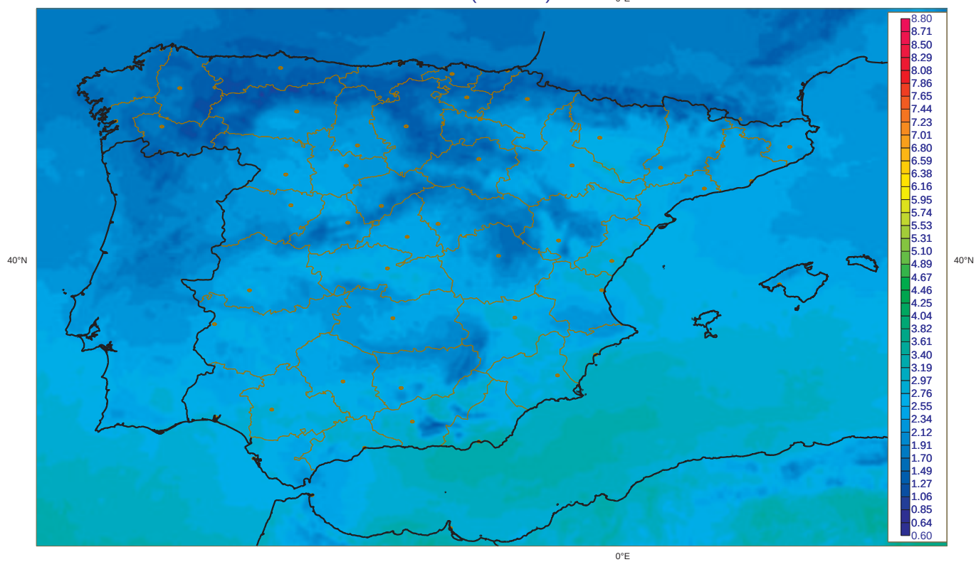
Irradiancia Global Febrero: Valores Minimos [1983-2005] (Kwh m-2 dia-1) SIS (CM-SAF)
