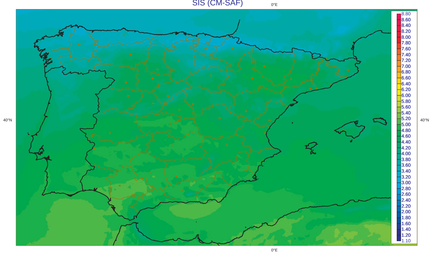
Irradiancia Global media Marzo [1983-2005] (Kwh m-2 dia-1) SIS (CM-SAF)
