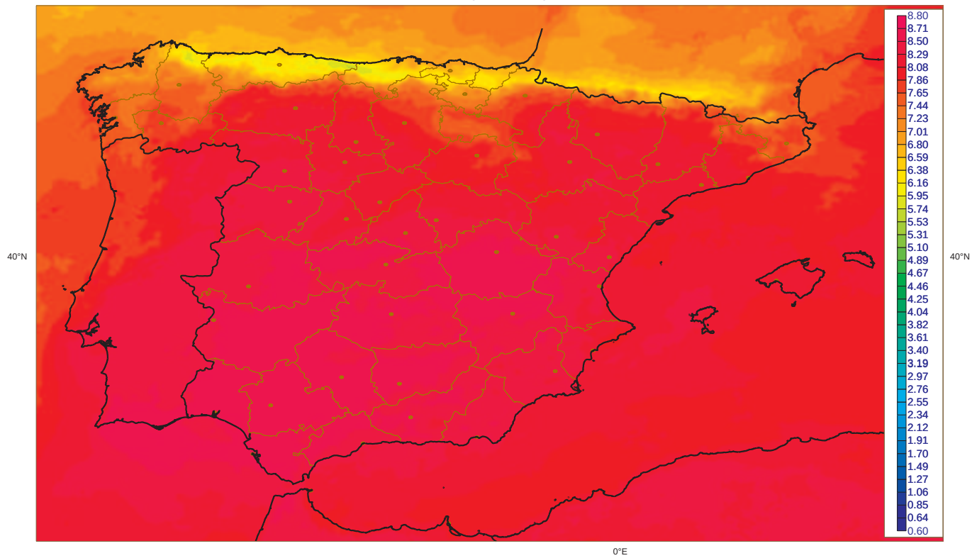
Irradiancia Global Junio: Valores Maximos [1983-2005] (Kwh m-2 dia-1) SIS (CM-SAF)
