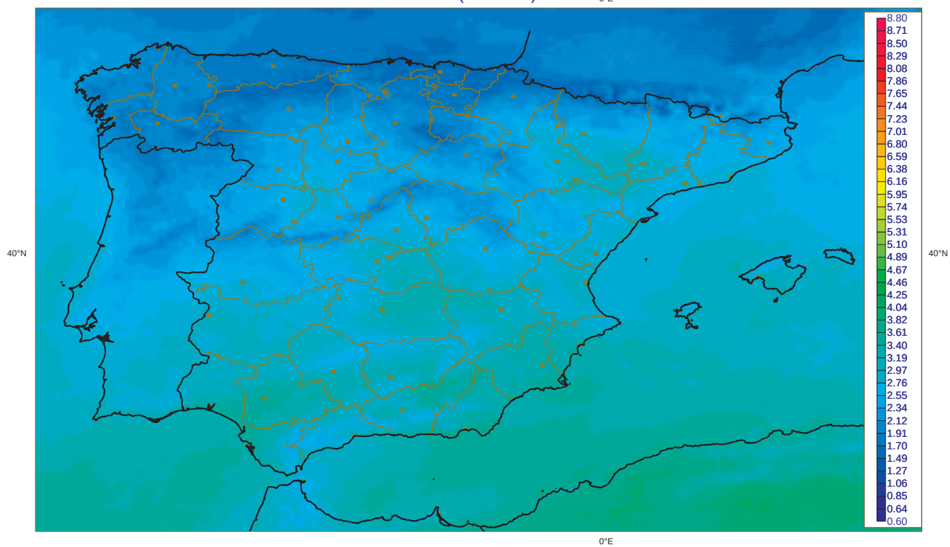
Irradiancia Global Octubre: Valores Minimos [1983-2005] (Kwh m-2 dia-1) SIS (CM-SAF)
