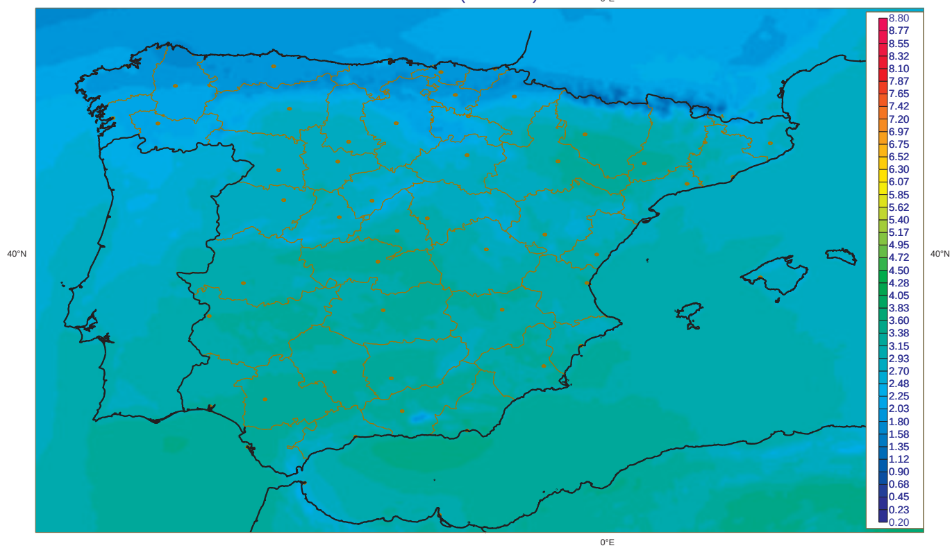
Irradiancia Directa media Marzo [1983-2005] (Kwh m-2 dia-1) SID (CM-SAF)
