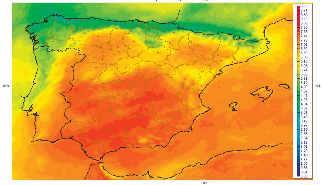
Irradiancia Global Julio: Valores Minimos [1983-2005] (Kwh m-2 dia-1) SIS (CM-SAF)
