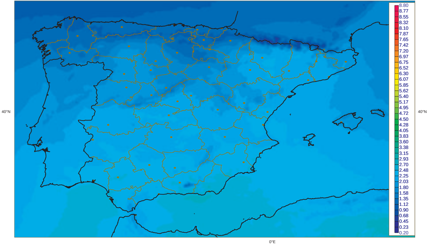
Irradiancia Directa media Febrero [1983-2005] (Kwh m-2 dia-1) SID (CM-SAF)
