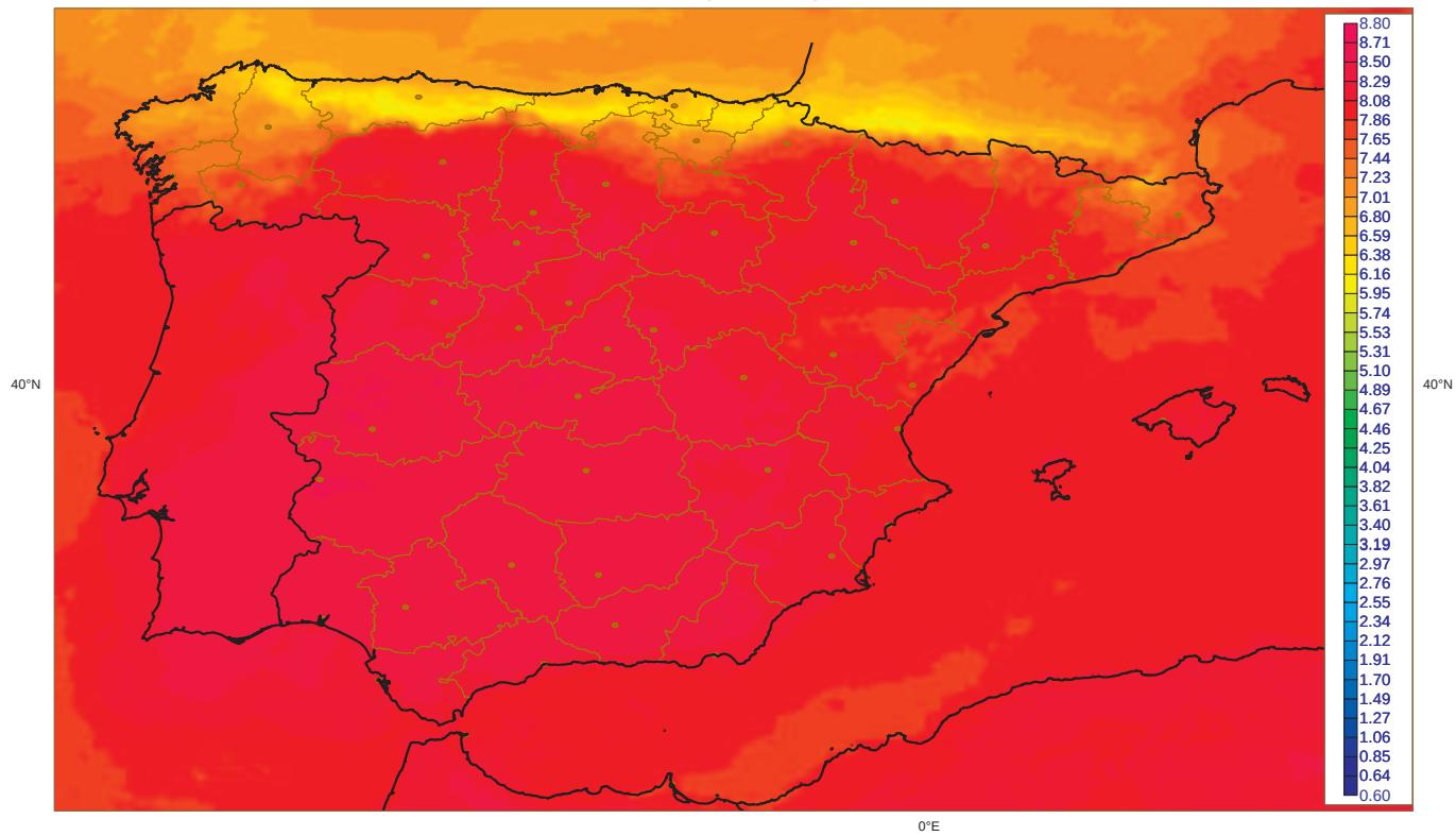
Irradiancia Global Julio: Valores Maximos [1983-2005] (Kwh m-2 dia-1) SIS (CM-SAF)
