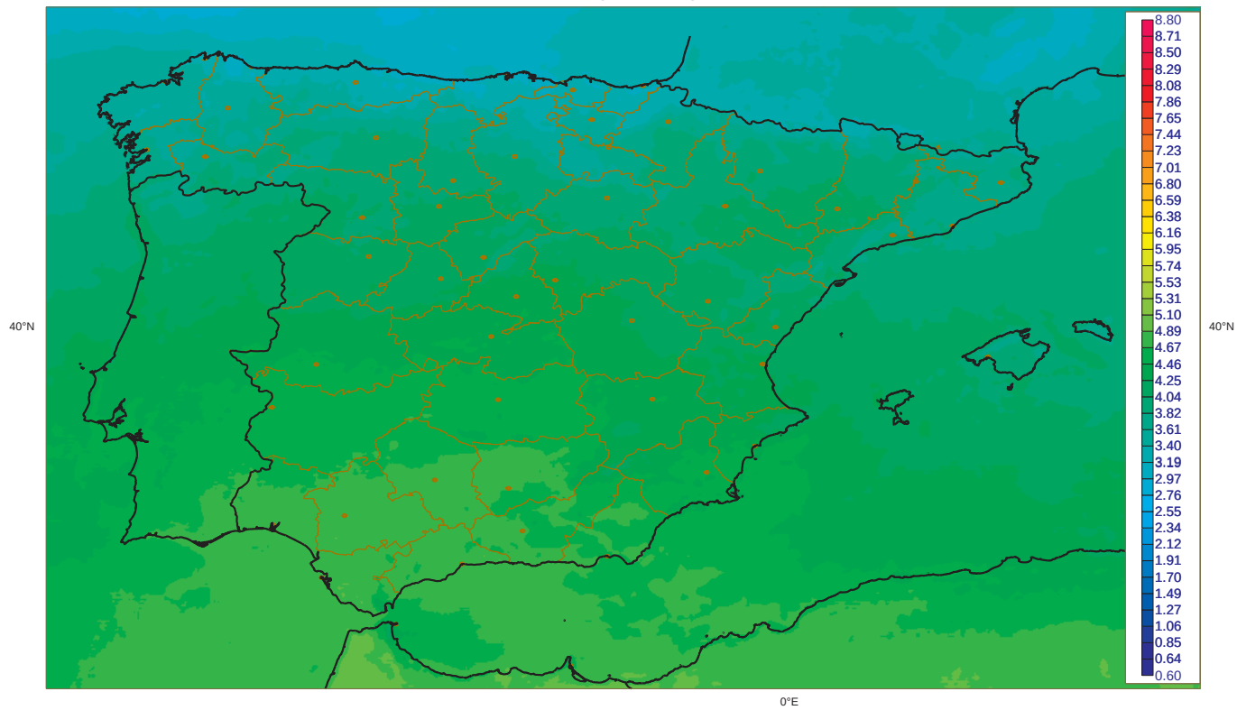
Irradiancia Global Octubre: Valores Maximos [1983-2005] (Kwh m-2 dia-1) SIS (CM-SAF)
