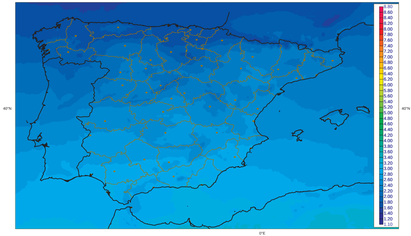
Irradiancia Global media Noviembre [1983-2005] (Kwh m-2 dia-1) SIS (CM-SAF)
