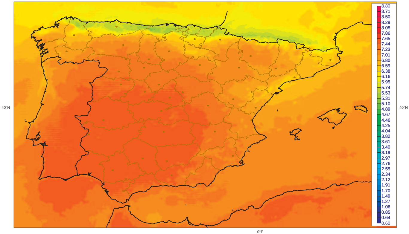
Irradiancia Global Agosto: Valores Maximos [1983-2005] (Kwh m-2 dia-1) SIS (CM-SAF)
