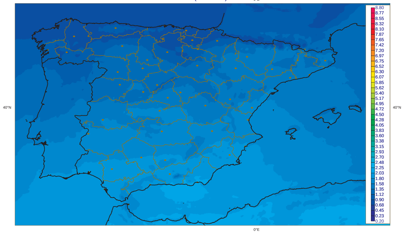
Irradiancia Directa media Noviembre [1983-2005] (Kwh m-2 dia-1) SID (CM-SAF)
