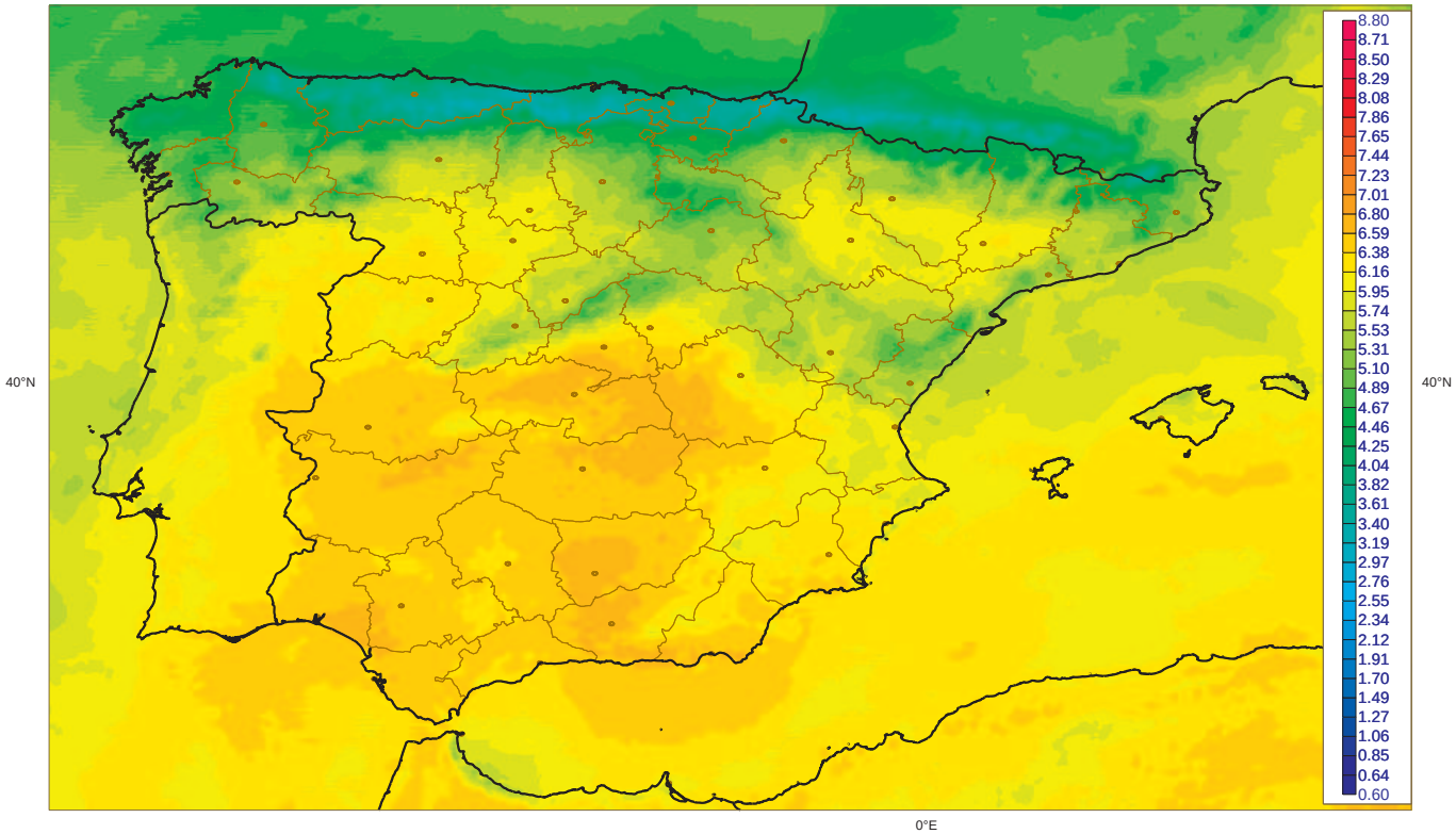
Irradiancia Global Agosto: Valores Minimos [1983-2005] (Kwh m-2 dia-1) SIS (CM-SAF)
