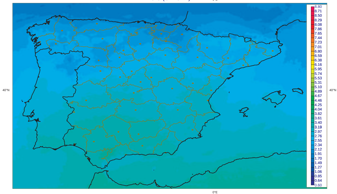
Irradiancia Global Enero: Valores Maximos [1983-2005] (Kwh m-2 dia-1) SIS (CM-SAF)
