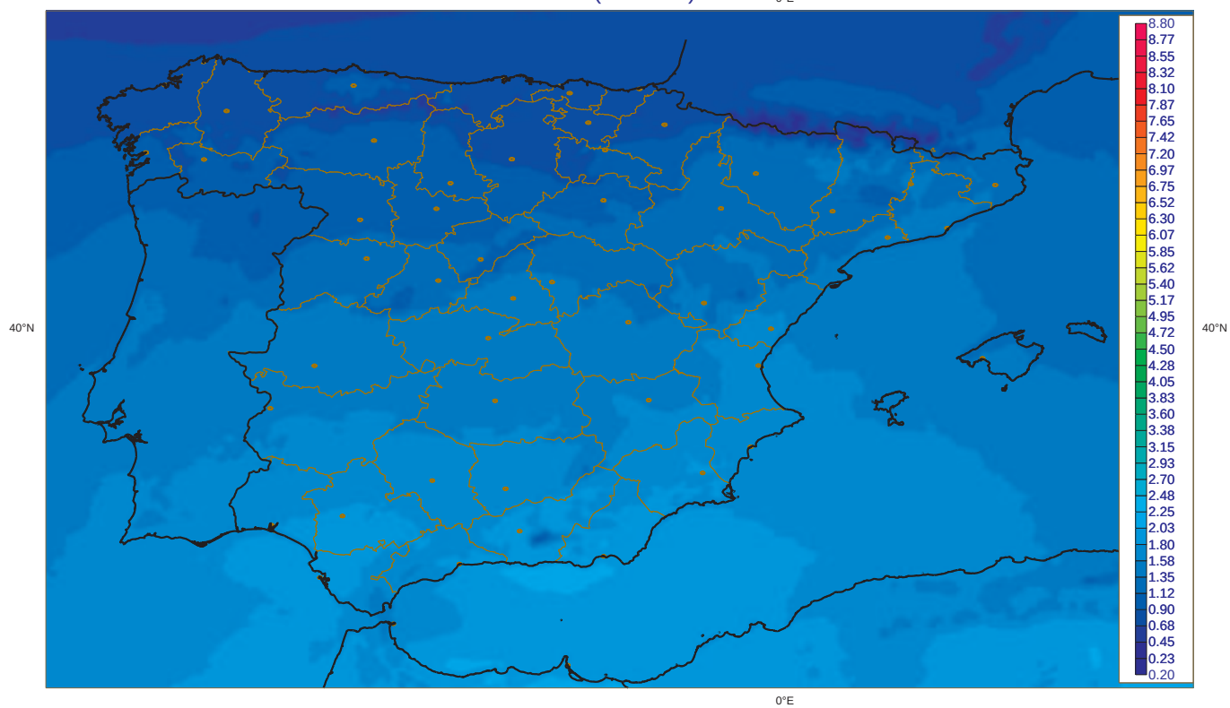
Irradiancia Directa media Enero [1983-2005] (Kwh m-2 dia-1) SID (CM-SAF)
