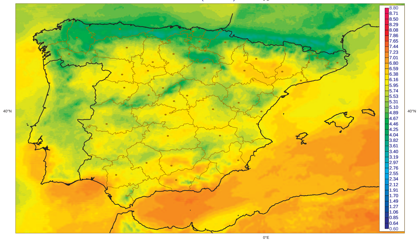
Irradiancia Global Junio: Valores Minimos [1983-2005] (Kwh m-2 dia-1) SIS (CM-SAF)
