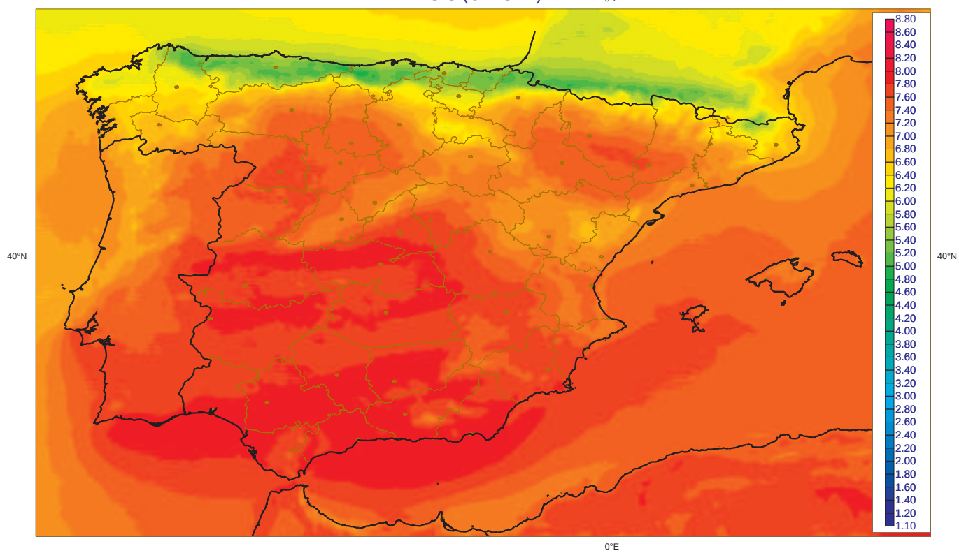
Irradiancia Global media Junio [1983-2005] (Kwh m-2 dia-1) SIS (CM-SAF)
