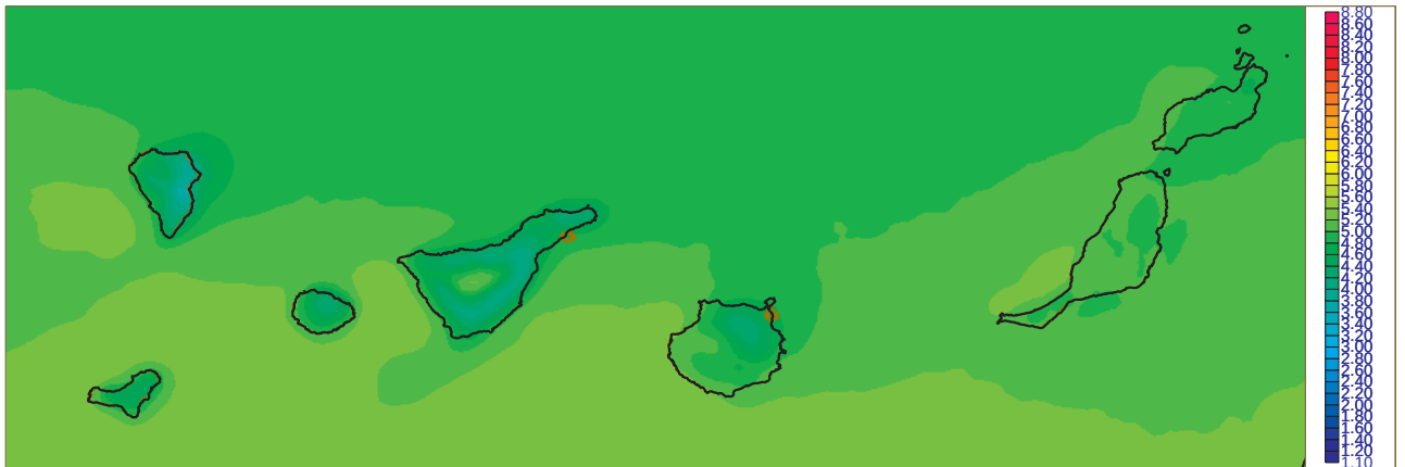
Irradiancia Global media Octubre [1983-2005] (Kwh m-2 dia-1) SIS (CM-SAF)
