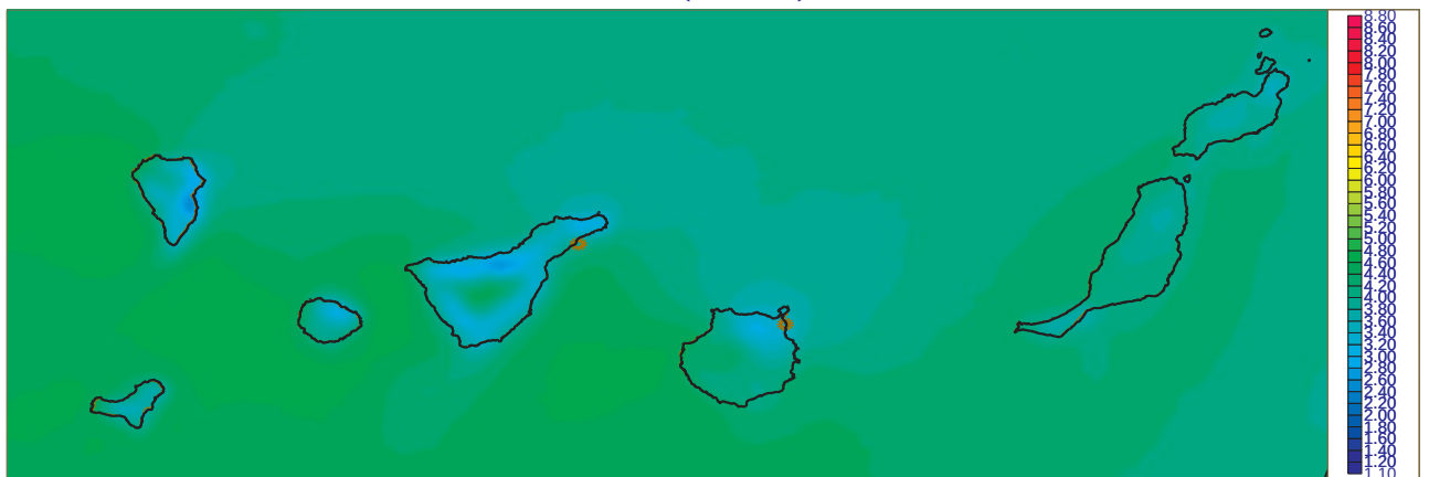
Irradiancia Directa media Septiembre [1983-2005] (Kwh m-2 dia-1) SID (CM-SAF)
