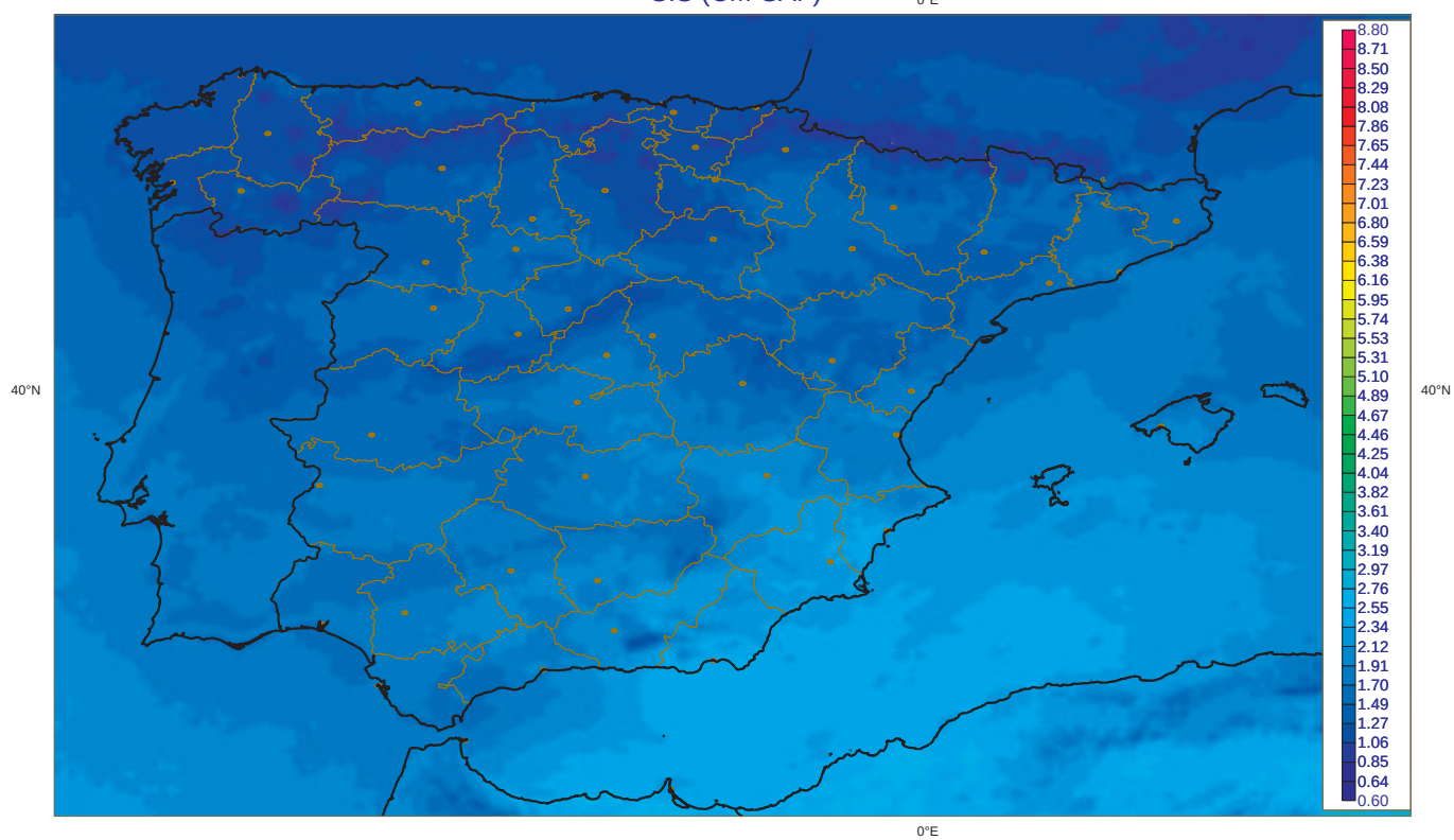
Irradiancia Global Enero: Valores Minimos [1983-2005] (Kwh m-2 dia-1) SIS (CM-SAF)
