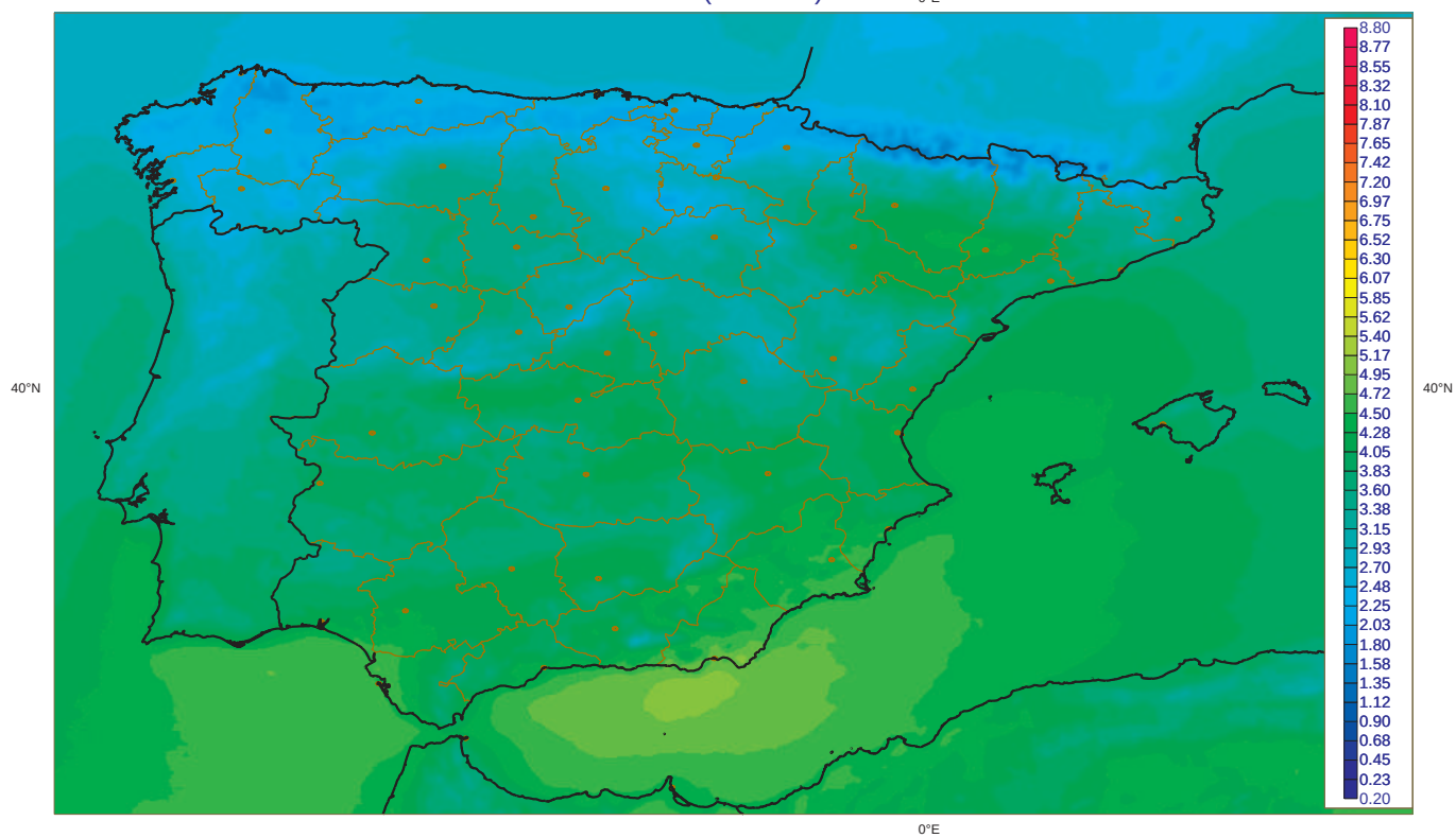
Irradiancia Directa media Abril [1983-2005] (Kwh m-2 dia-1) SID (CM-SAF)
