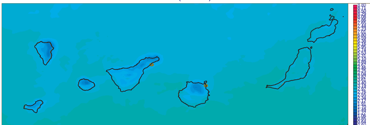
Irradiancia Global : Valores Minimos [1983-2005] (Kwh m-2 dia-1) SIS (CM-SAF)
