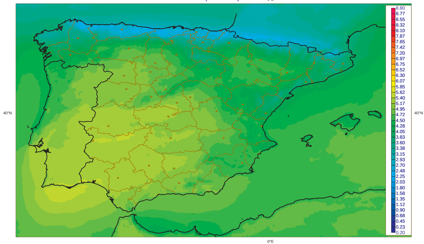
Irradiancia Directa media Agosto [1983-2005] (Kwh m-2 dia-1) SID (CM-SAF)
