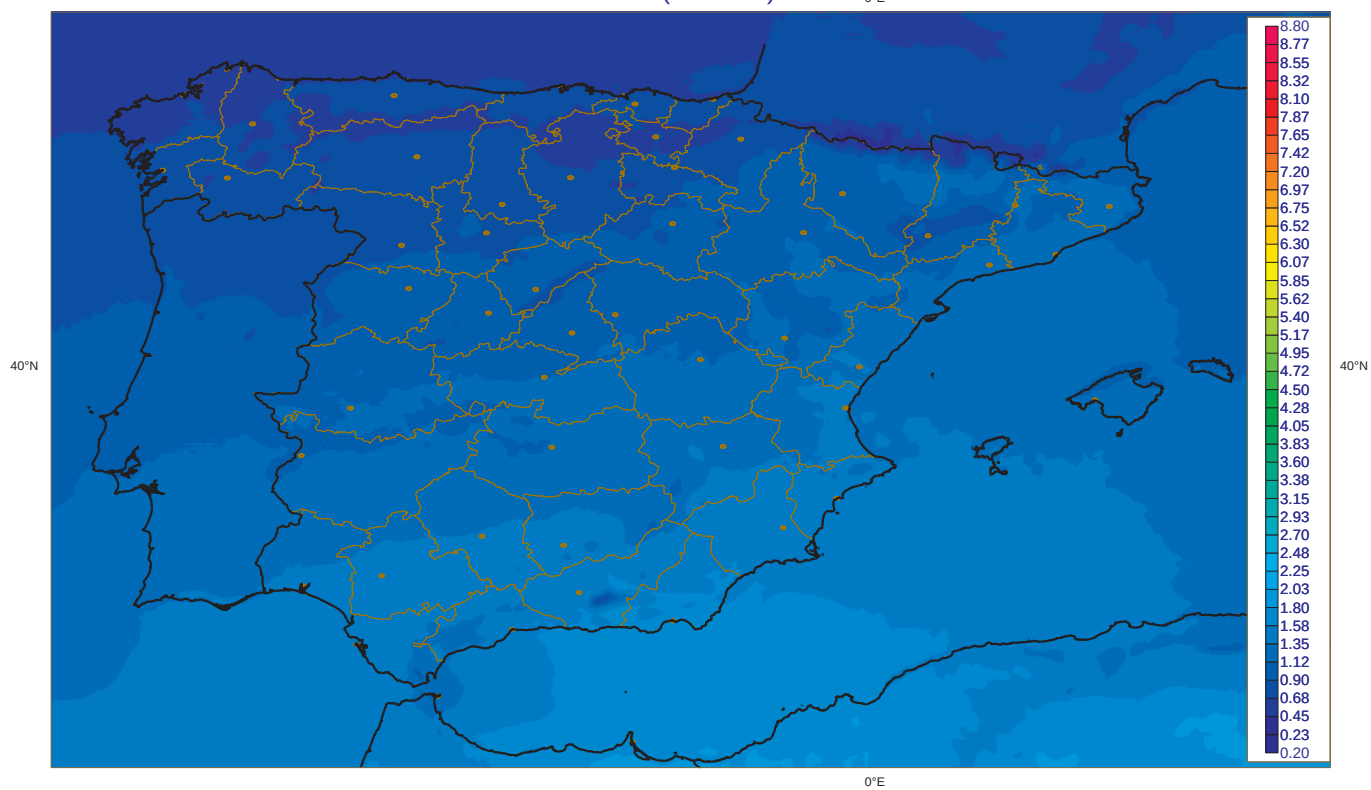
Irradiancia Directa media Diciembre [1983-2005] (Kwh m-2 dia-1) SID (CM-SAF)
