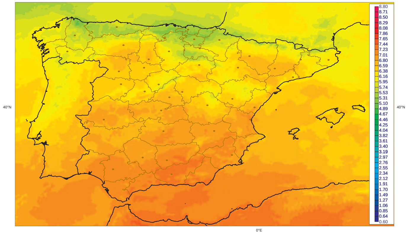
Irradiancia Global Abril: Valores Maximos [1983-2005] (Kwh m-2 dia-1) SIS (CM-SAF)
