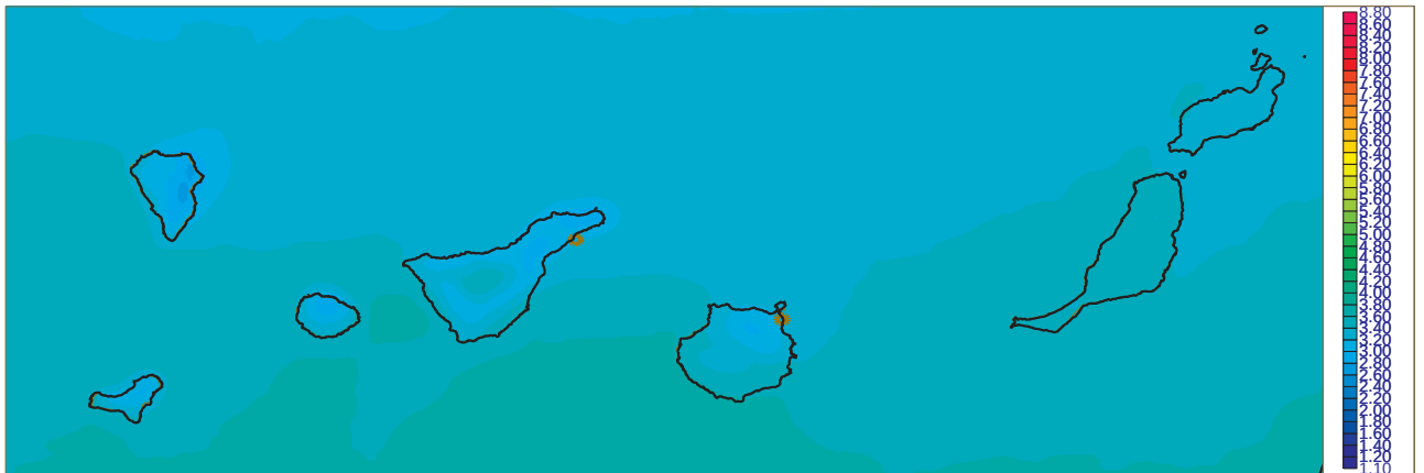
Irradiancia Global media Diciembre [1983-2005] (Kwh m-2 dia-1) SIS (CM-SAF)
