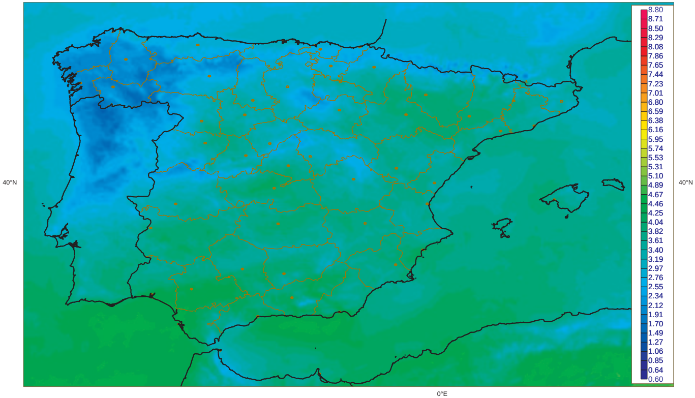
Irradiancia Global Marzo: Valores Minimos [1983-2005] (Kwh m-2 dia-1) SIS (CM-SAF)
