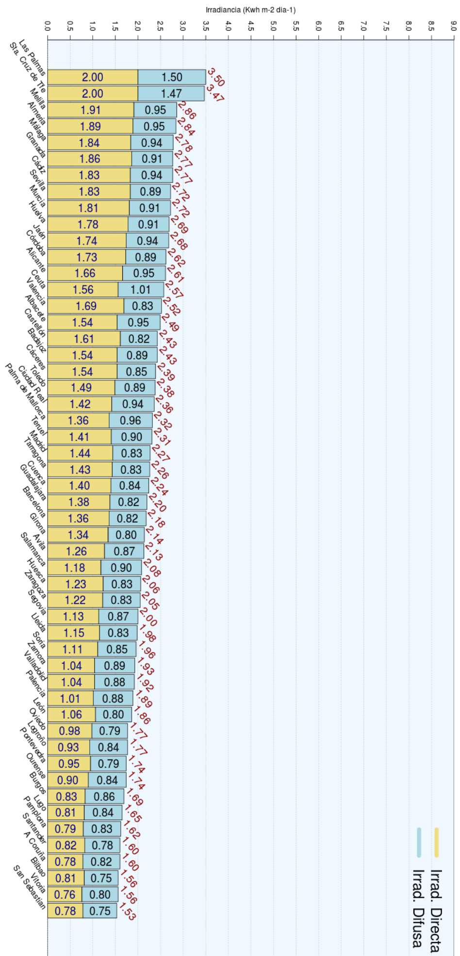
Irradiancia global media diaria, Mes: Enero [1983-2005]
