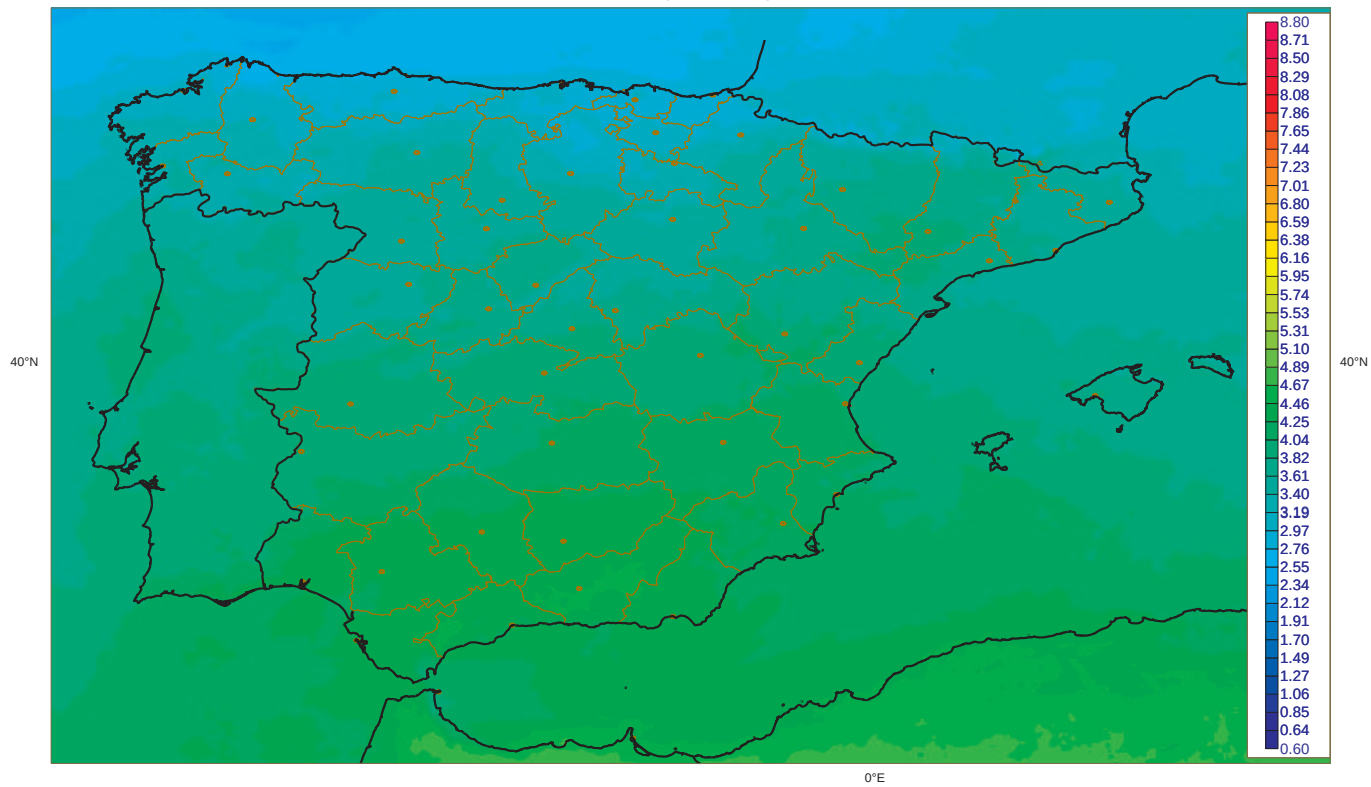
Irradiancia Global Febrero: Valores Maximos [1983-2005] (Kwh m-2 dia-1) SIS (CM-SAF)
