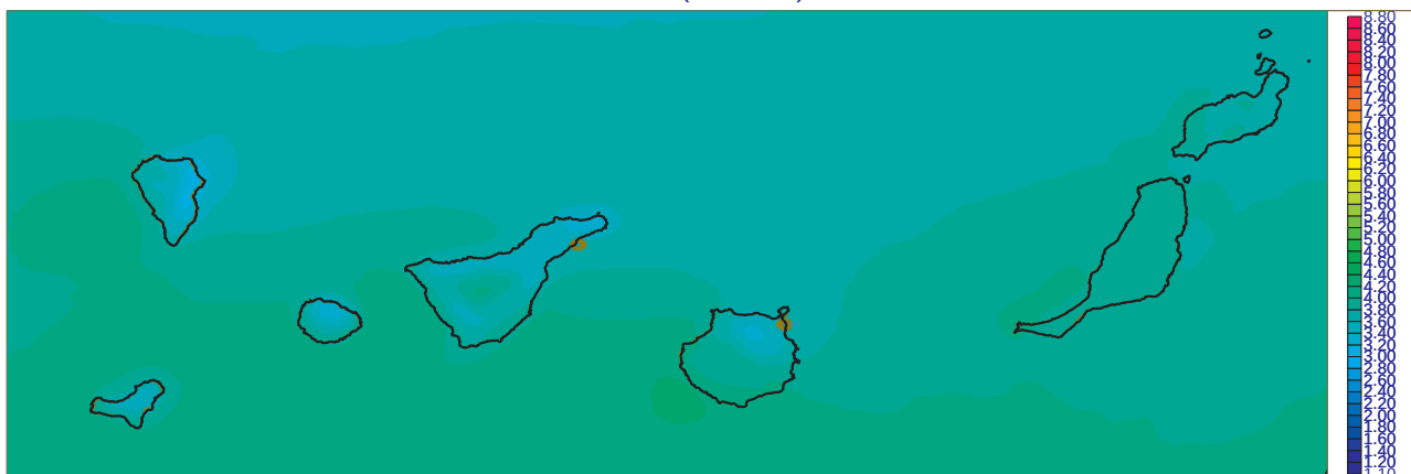
Irradiancia Global media en Invierno (Dic, Ene, Feb)[1983-2005] (Kwh m-2 dia-1) SIS (CM-SAF)
