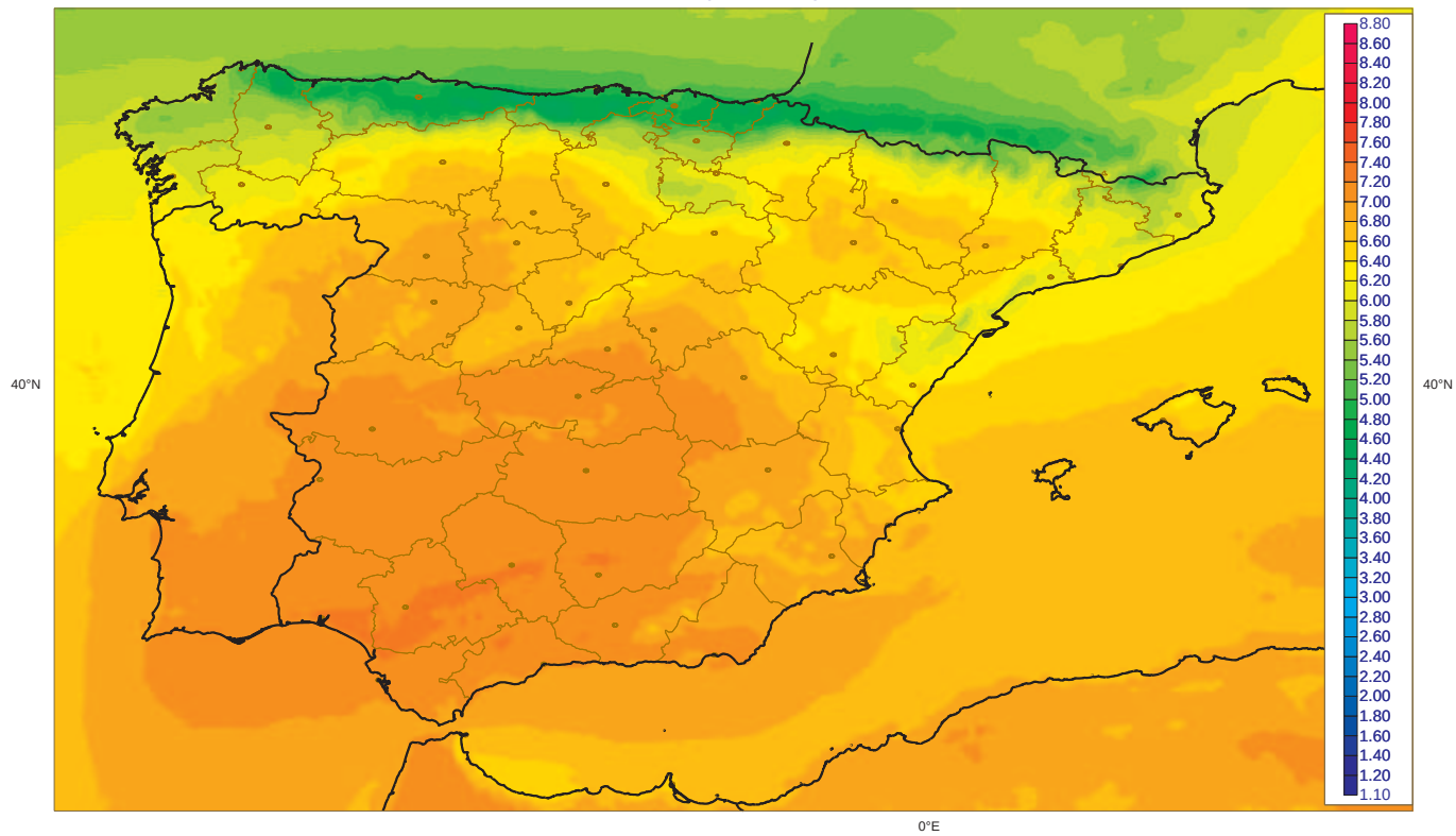
Irradiancia Global media Agosto [1983-2005] (Kwh m-2 dia-1) SIS (CM-SAF)
