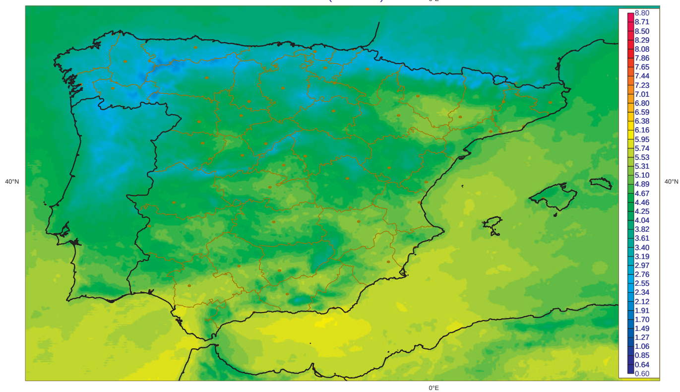
Irradiancia Global Abril: Valores Minimos [1983-2005] (Kwh m-2 dia-1) SIS (CM-SAF)
