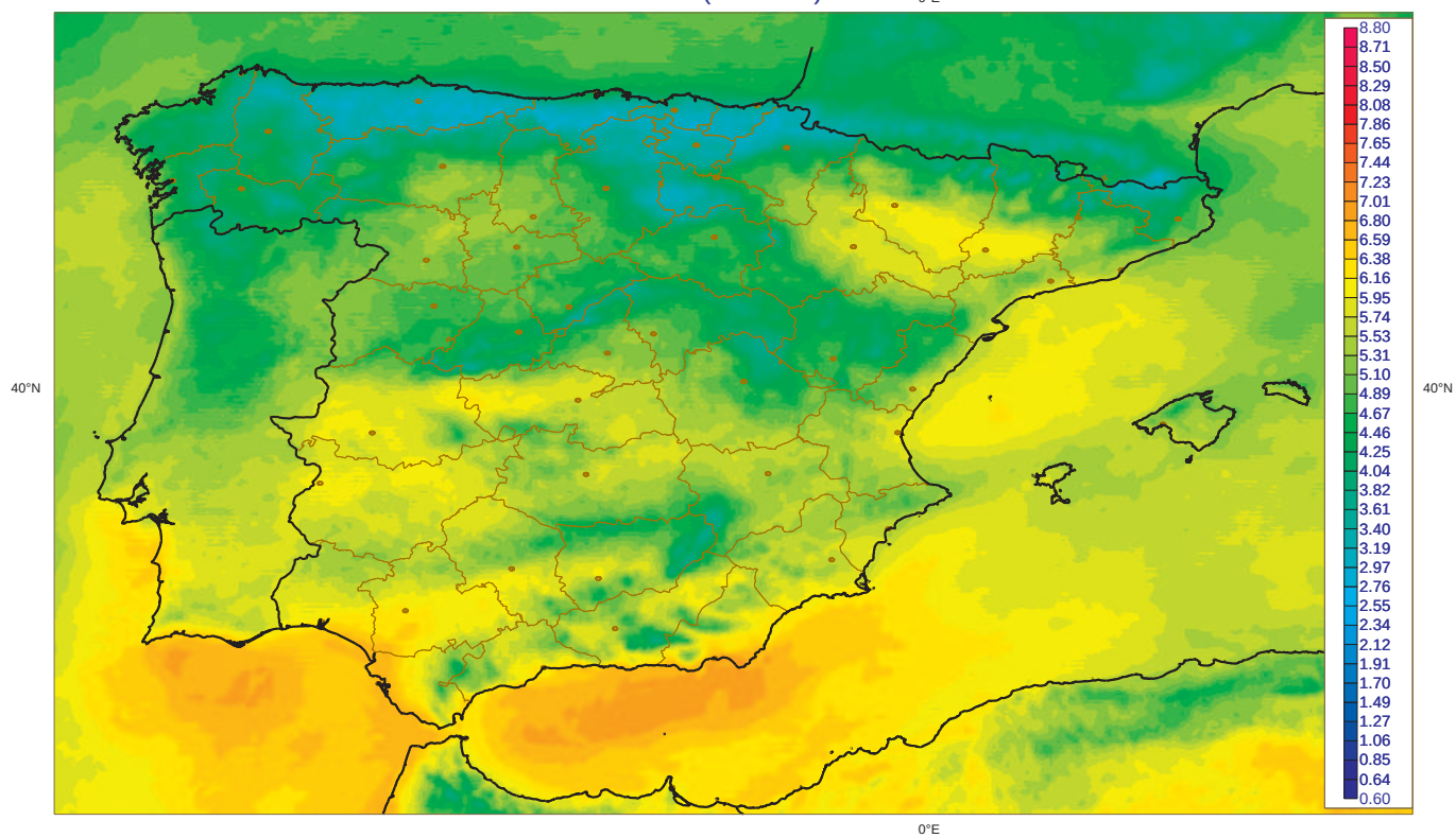
Irradiancia Global Mayo: Valores Minimos [1983-2005] (Kwh m-2 dia-1) SIS (CM-SAF)
