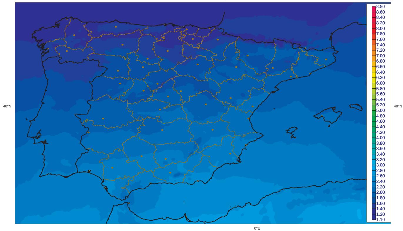
Irradiancia Global media Diciembre [1983-2005] (Kwh m-2 dia-1) SIS (CM-SAF)
