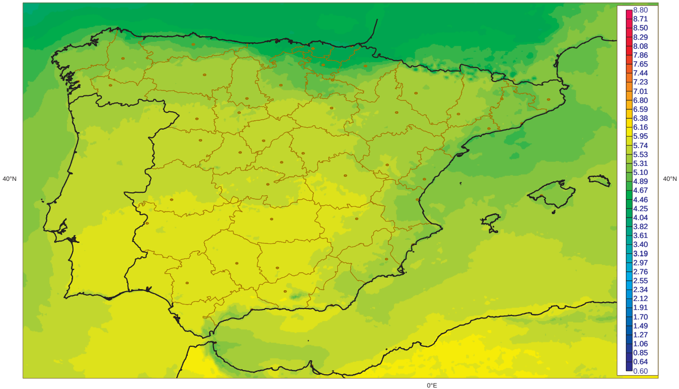
Irradiancia Global Marzo: Valores Maximos [1983-2005] (Kwh m-2 dia-1) SIS (CM-SAF)
