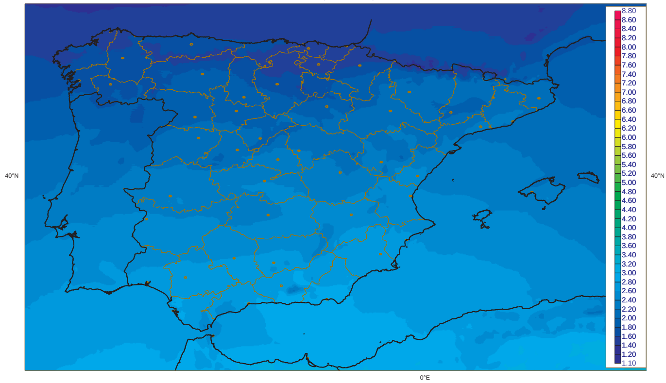
Irradiancia Global media Enero [1983-2005] (Kwh m-2 dia-1) SIS (CM-SAF)
