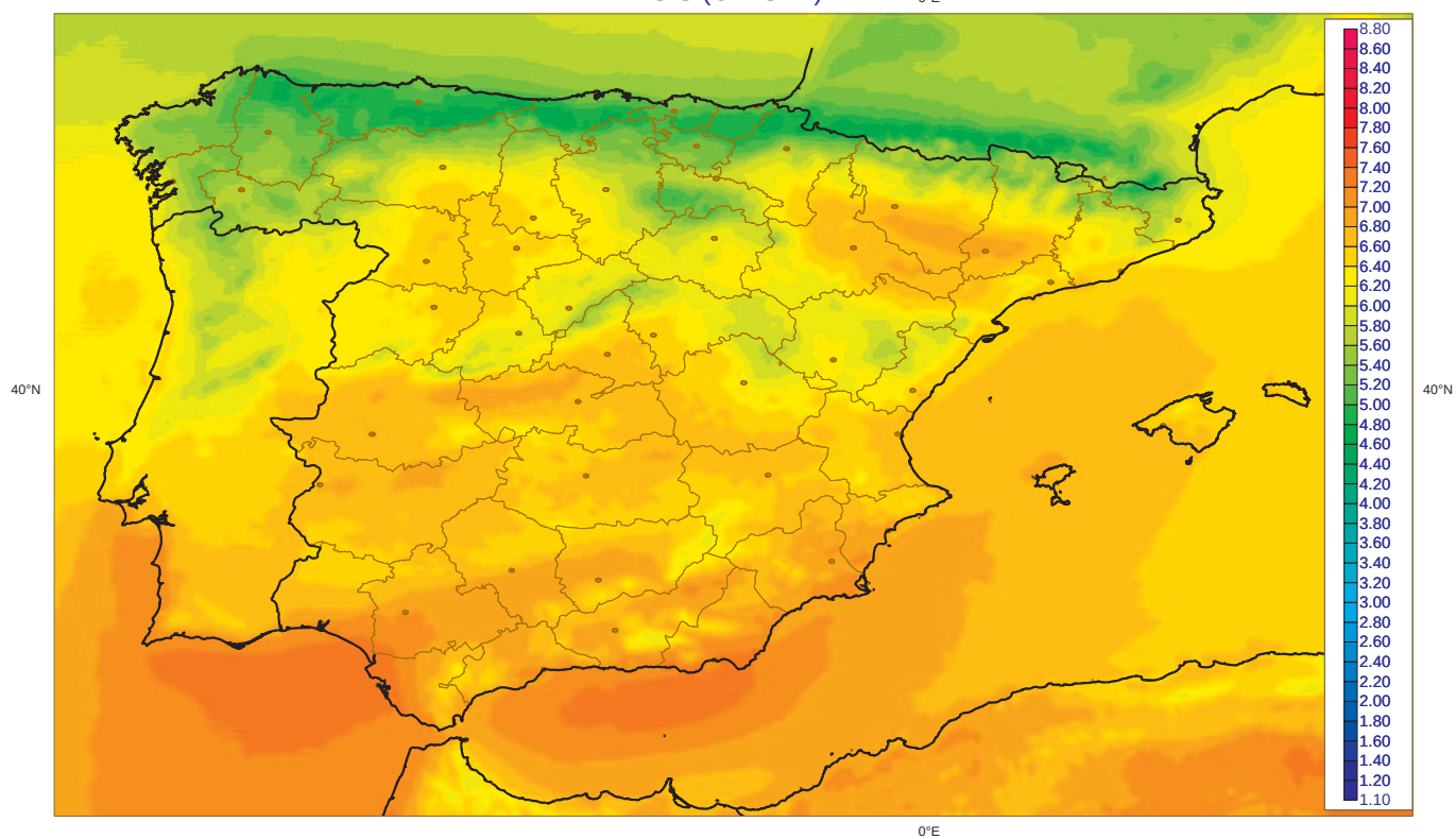
Irradiancia Global media Mayo [1983-2005] (Kwh m-2 dia-1) SIS (CM-SAF)
