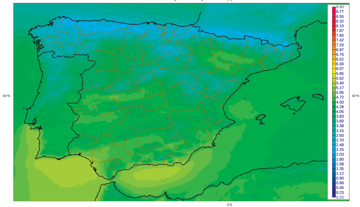
Irradiancia Directa media Mayo [1983-2005] (Kwh m-2 dia-1) SID (CM-SAF)
