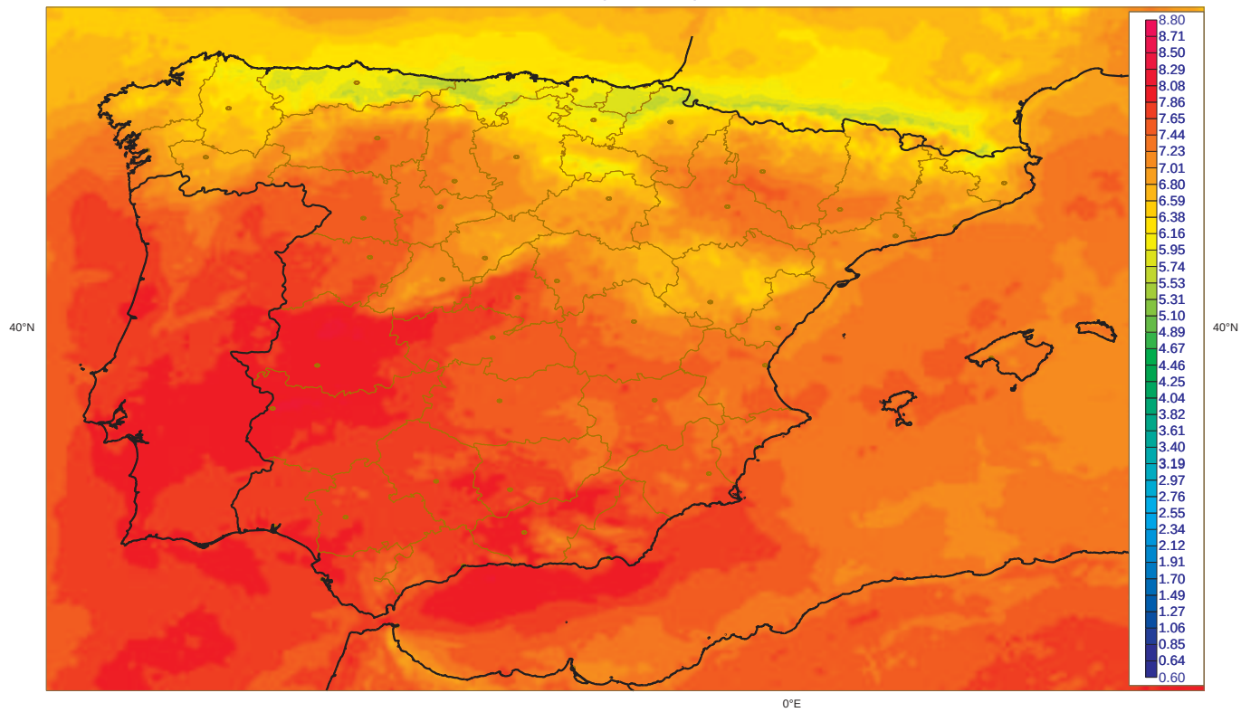
Irradiancia Global Mayo: Valores Maximos [1983-2005] (Kwh m-2 dia-1) SIS (CM-SAF)
