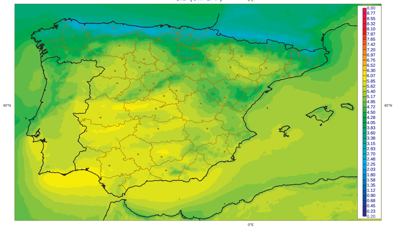
Irradiancia Directa media Junio [1983-2005] (Kwh m-2 dia-1) SID (CM-SAF)
