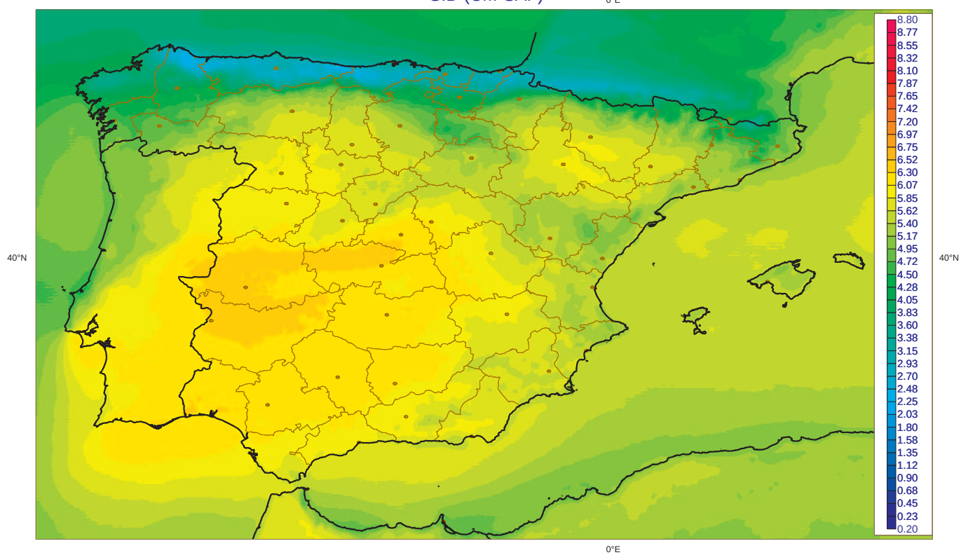
Irradiancia Directa media Julio [1983-2005] (Kwh m-2 dia-1) SID (CM-SAF)
