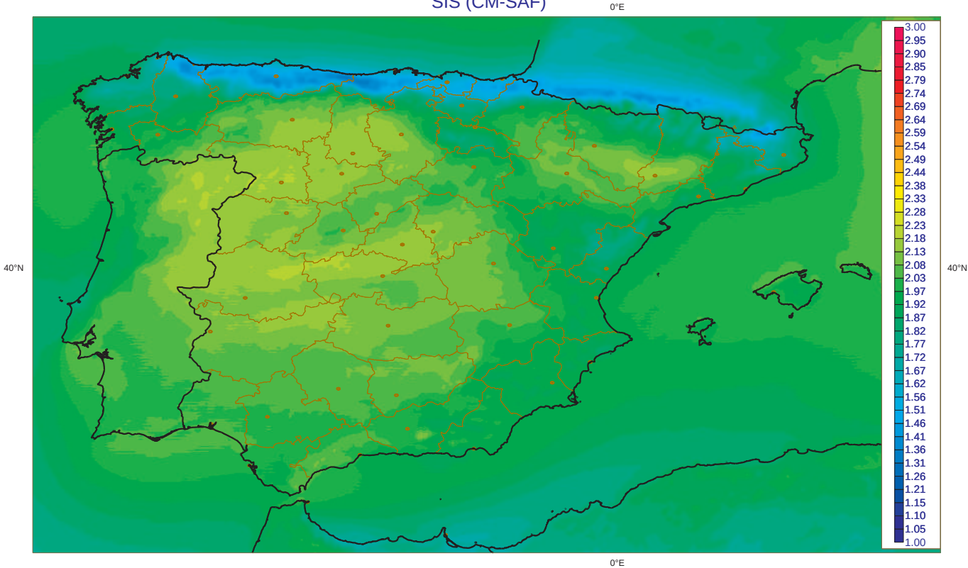
Irradiancia Global : Variabilidad Interanual (Desv. Estandar) [1983-2005] (Kwh m-2 dia-1) SIS (CM-SAF)
