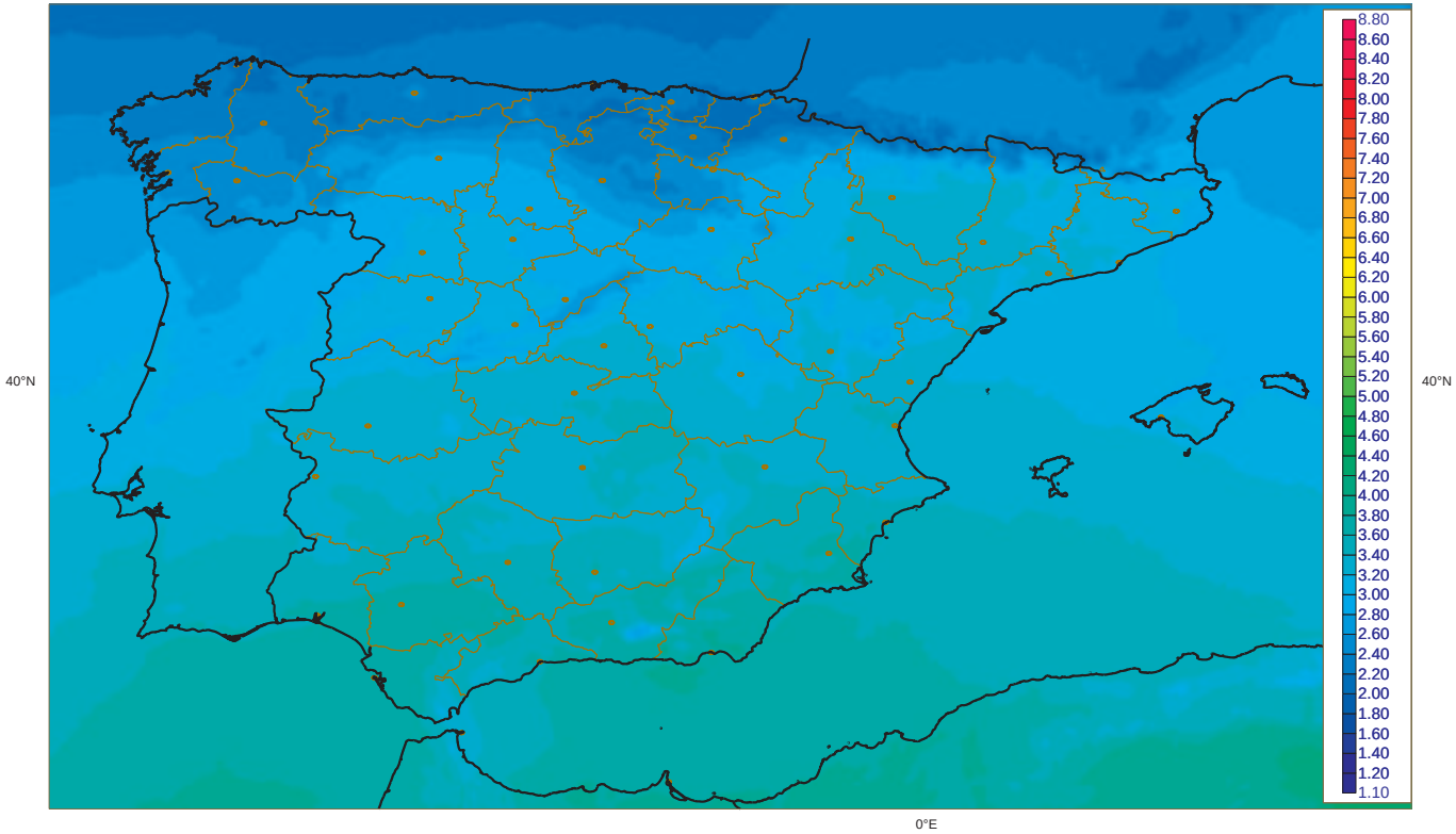
Irradiancia Global media Febrero [1983-2005] (Kwh m-2 dia-1) SIS (CM-SAF)
