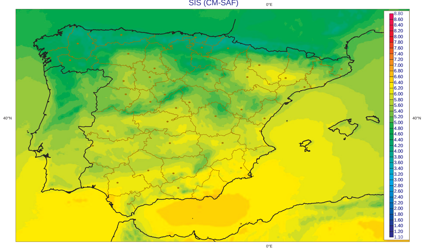
Irradiancia Global media Abril [1983-2005] (Kwh m-2 dia-1) SIS (CM-SAF)
