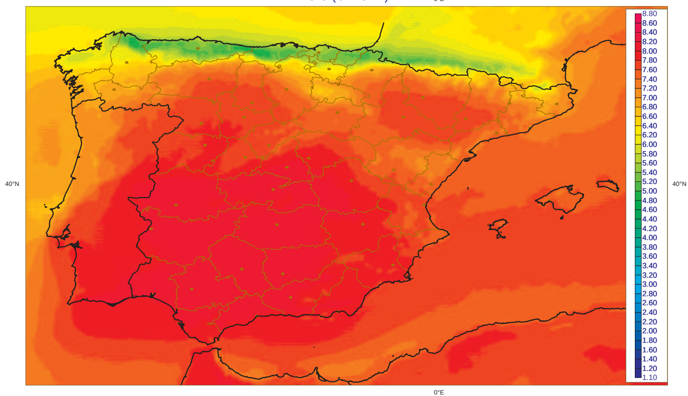
Irradiancia Global media Julio [1983-2005] (Kwh m-2 dia-1) SIS (CM-SAF)
