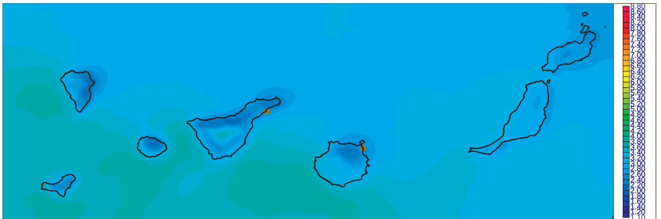
Irradiancia Directa media Marzo [1983-2005] (Kwh m-2 dia-1) SID (CM-SAF)
